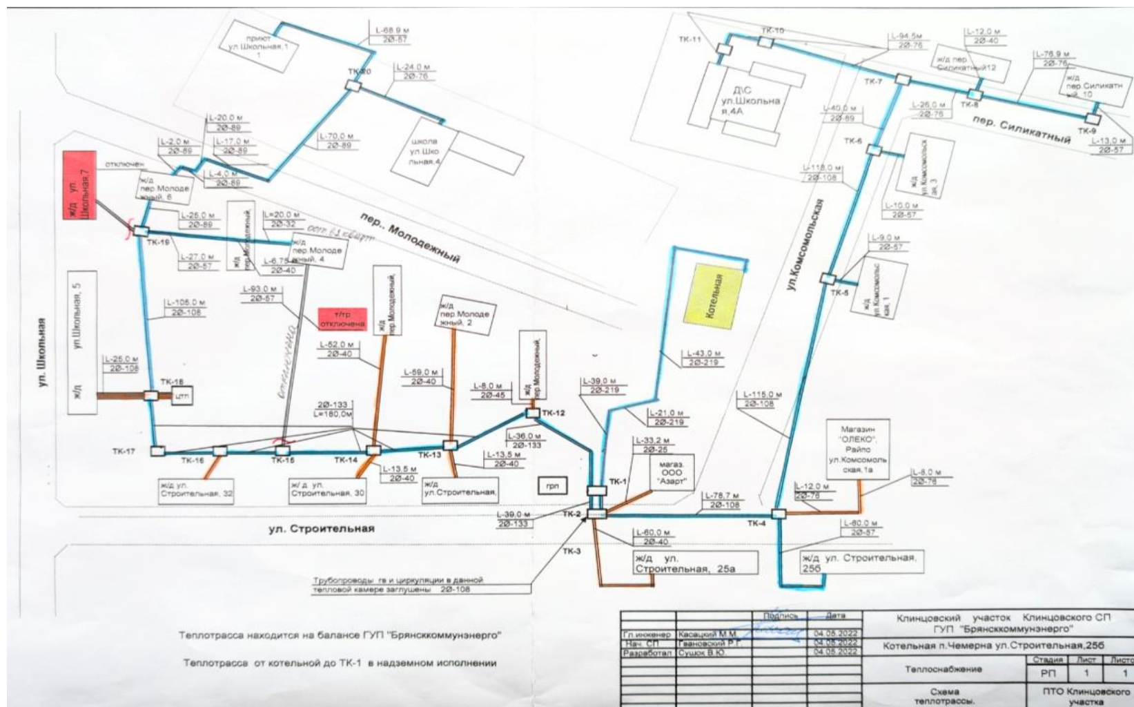
Схема 1. Тепловые сети котельной ГУП «Брянсккоммунэнерго» п. Черна, кот. ул. Строительная, 256
