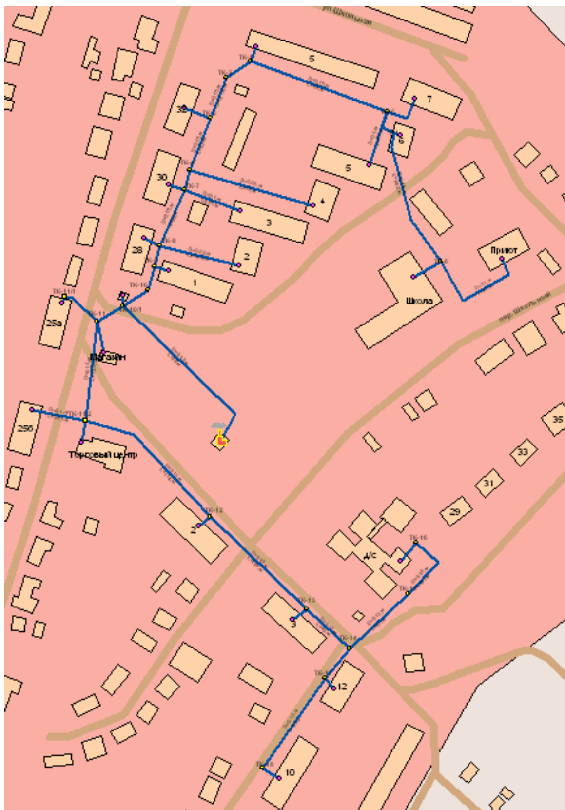
Рисунок 3 - Схема теплоснабжения поселка Чемерна
