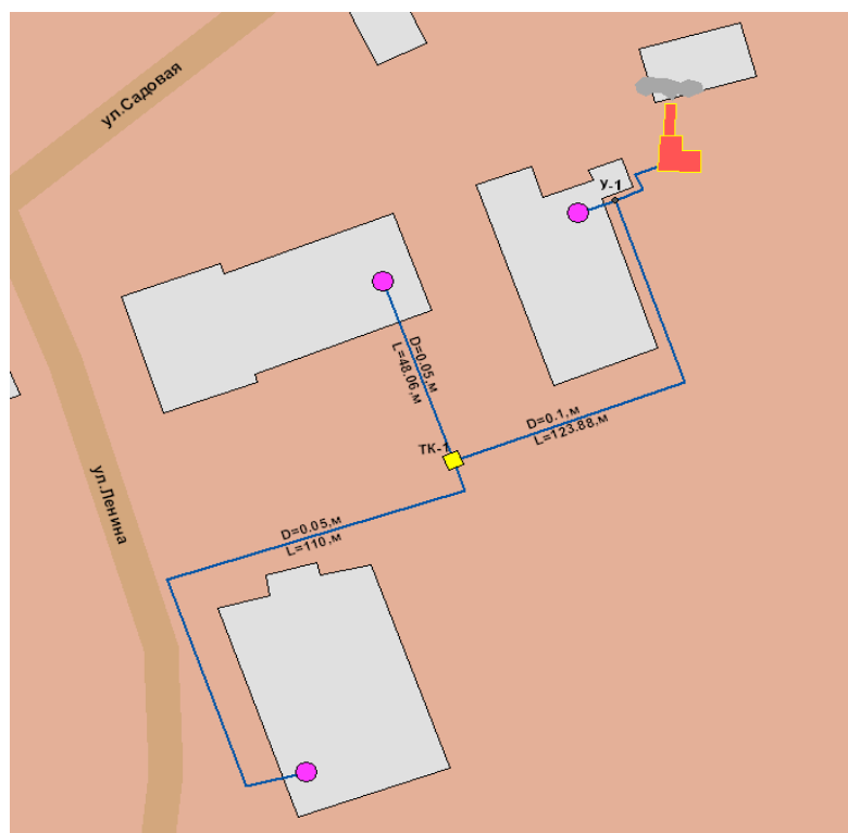
Рисунок 2 – Схема теплоснабжения села Смолевичи
