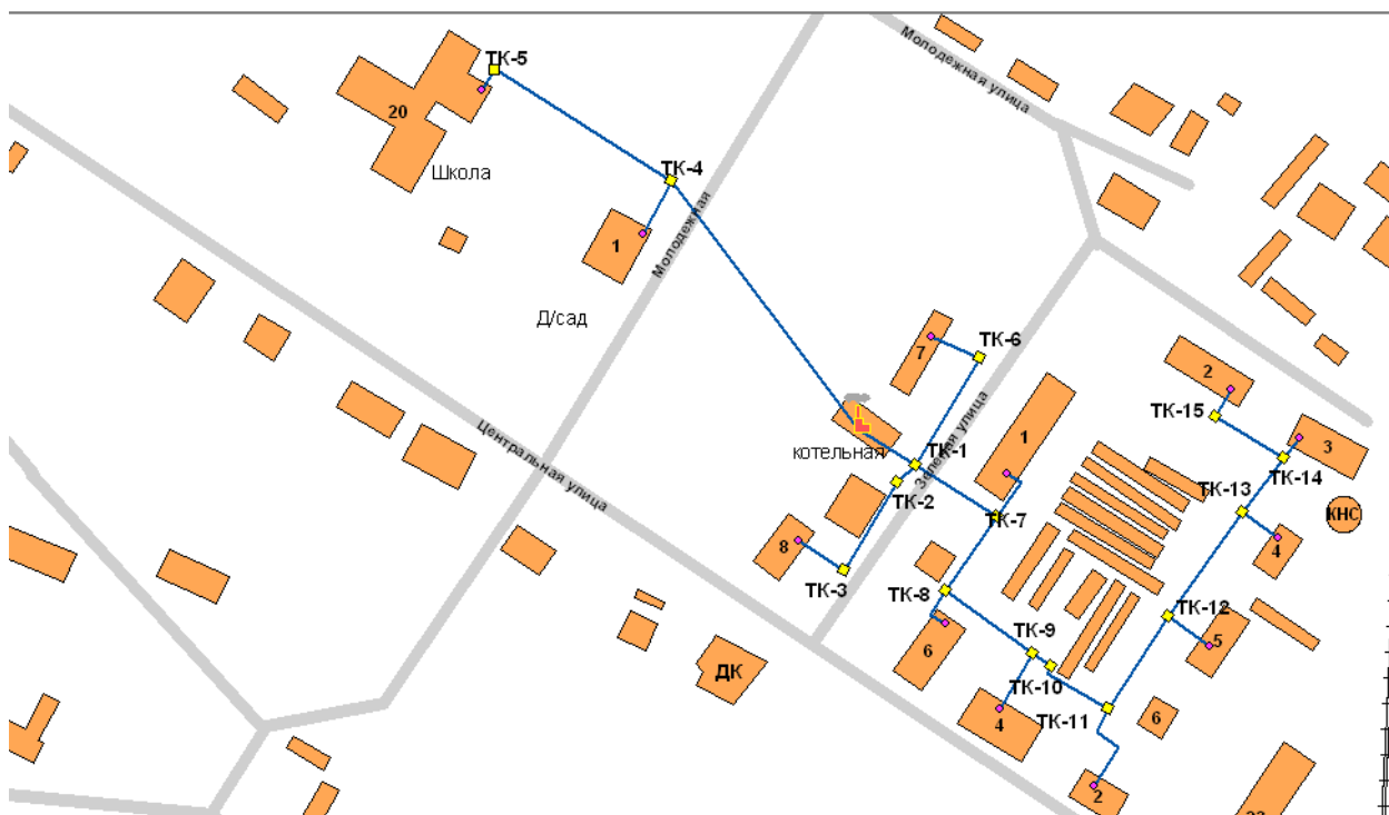
Рисунок 4 – Схема теплоснабжения Первомайского сельского поселения (п. Первое Мая)
