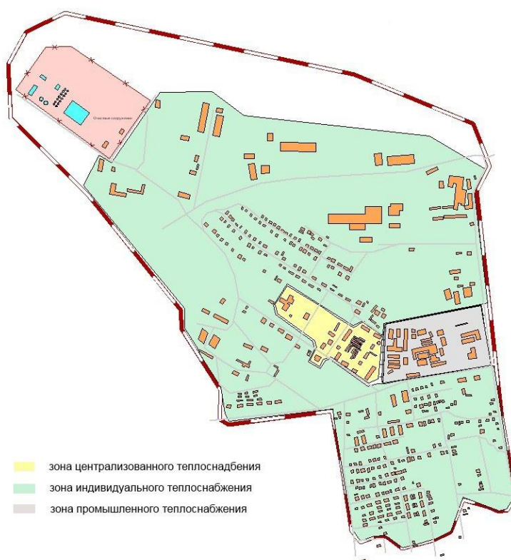
Рисунок 5 – Зоны теплоснабжения Первомайского сельского поселения
