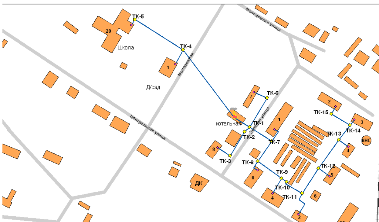
Рисунок 2 – Схема теплоснабжения Первомайского сельского поселения (п. Первое Мая)
