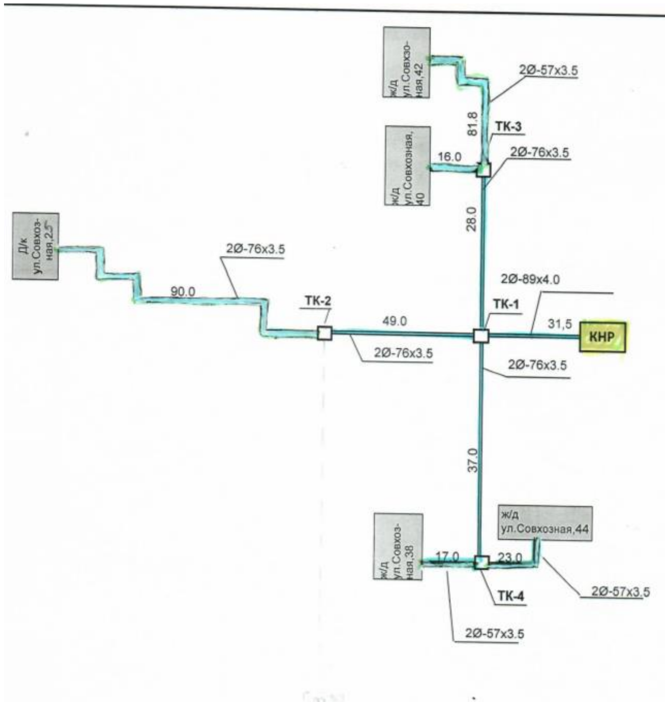
Карта-схема 1 Тепловые сети в зонах действия котельной с. Коржовка-Голубовка, КНР, ул. Совхозная.
