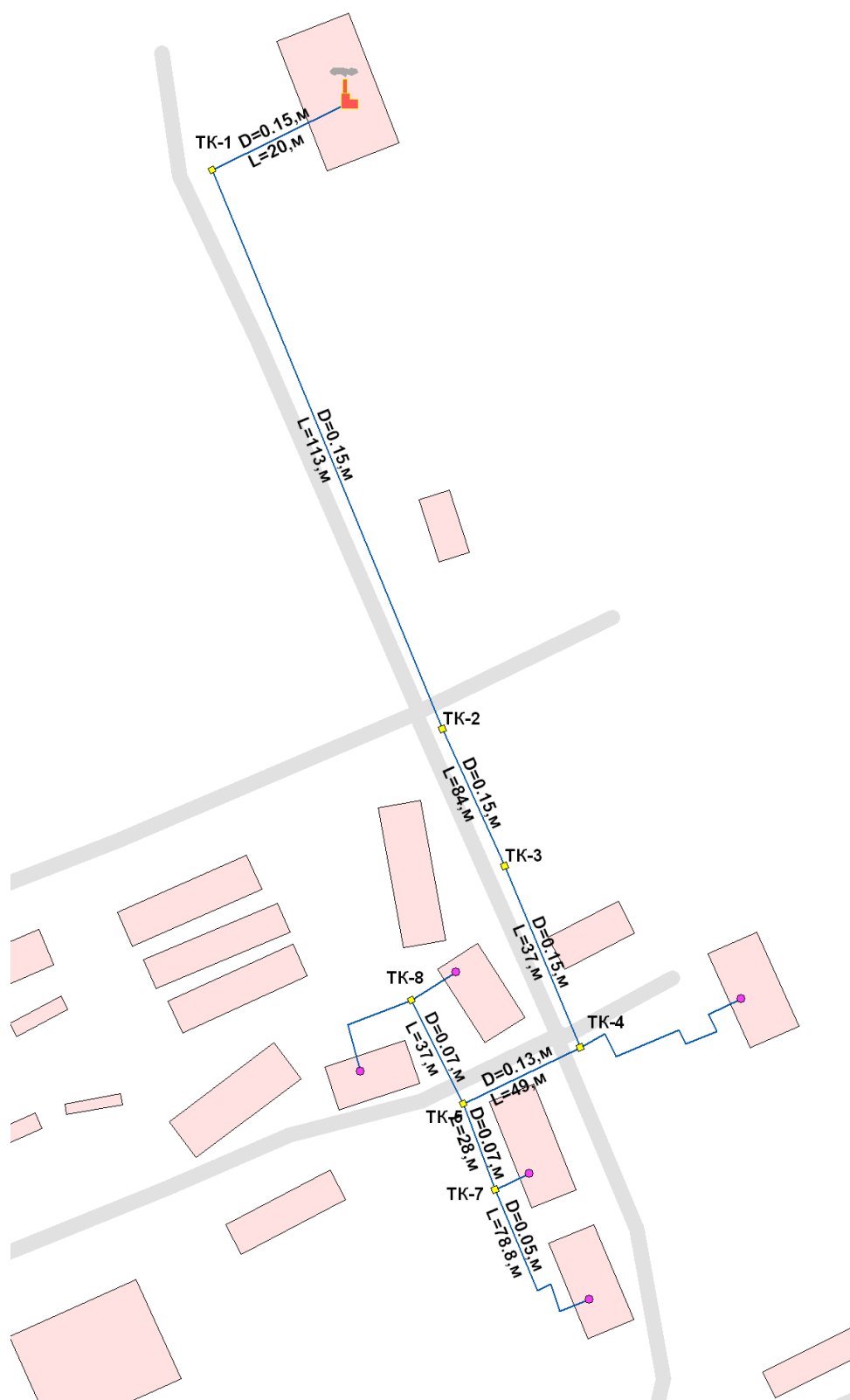
Рисунок 3 - Схема тепловой сети системы отопления от котельной с. Коржовка-Голубовка.
