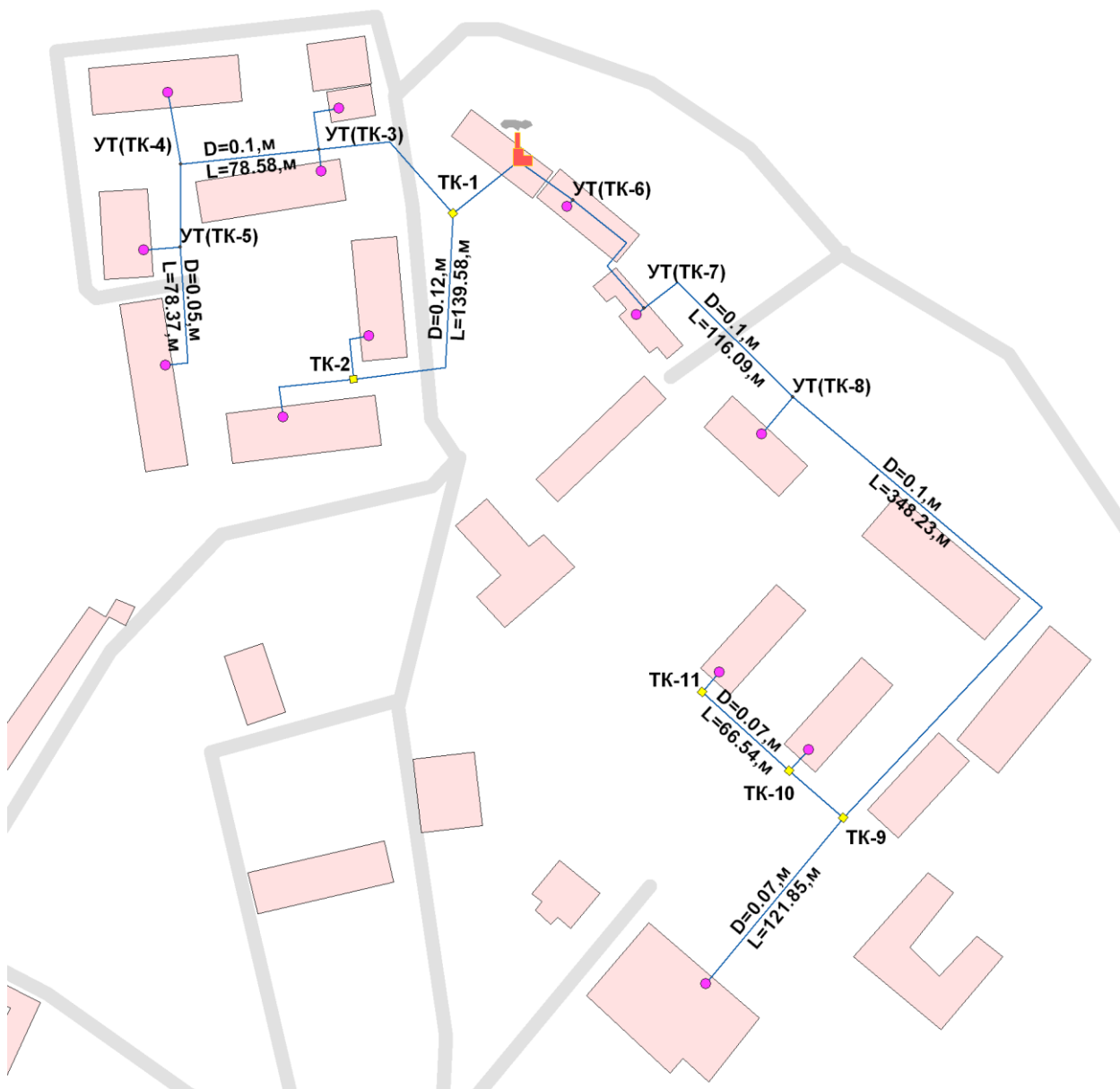
Рисунок 4 - Схема тепловой сети системы отопления от котельной с. Затишье
